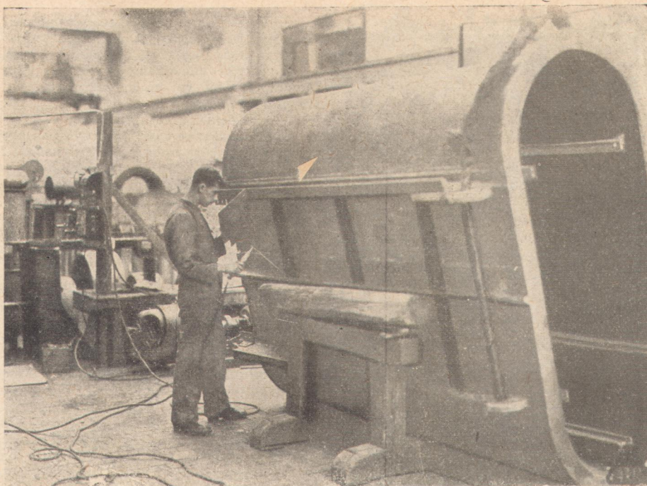
Зварюють „кожух“ трансформаторного котла
