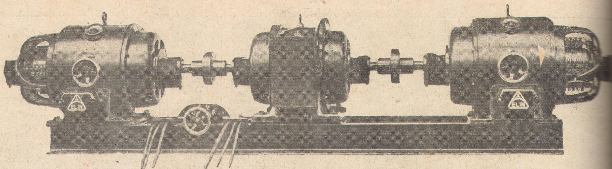
Подвійний агрегат для електрозварювання
