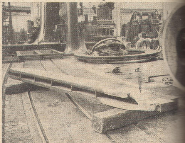
Зразок роботи електричною зваркою
