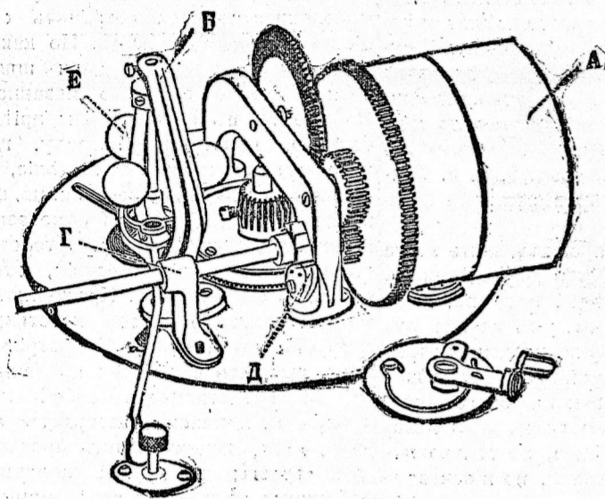
Внутренній механизмъ новаго двухпружиннаго граммофона. Внутренній механизмъ новаго трехпружиннаго граммофона.
