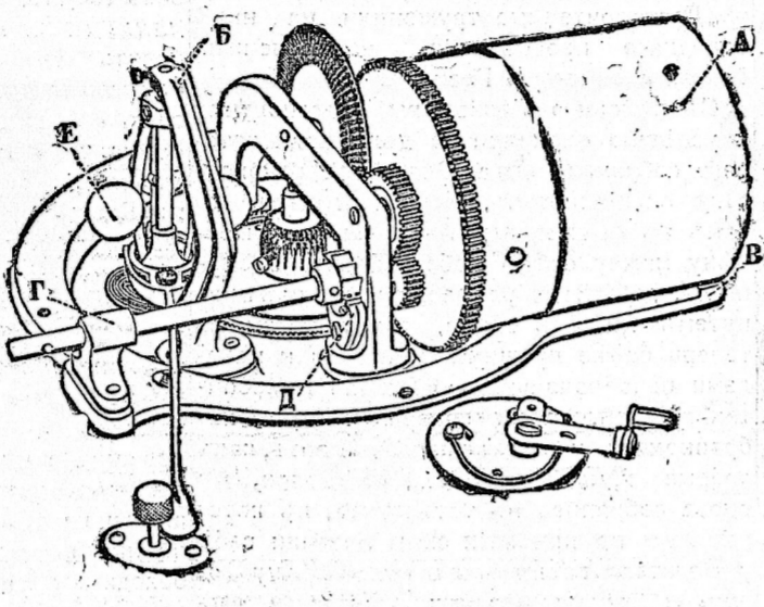
Внутренній механизмъ новаго двухпружиннаго граммофона. Внутренній механизмъ новаго трехпружиннаго граммофона.
